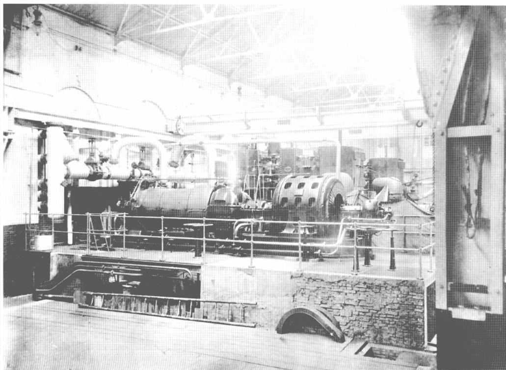
清光绪十三年（1887年）安装在新中央电站的国内第一台 800 千瓦派生斯汽轮发电机组
