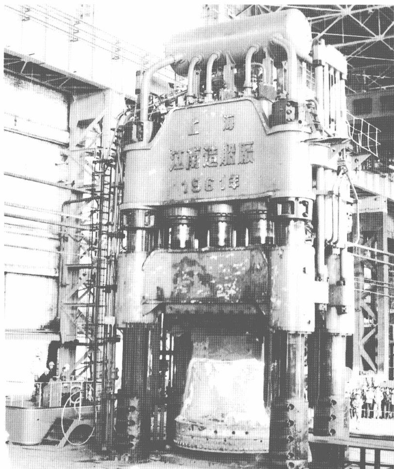
1961年以 上海江南造船厂和 上海重型机器厂为主制造的 12000吨水压机
