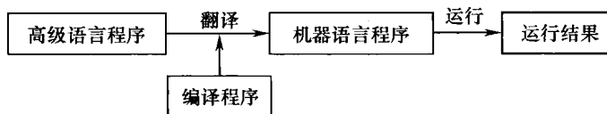
图 1-3 编译过程
