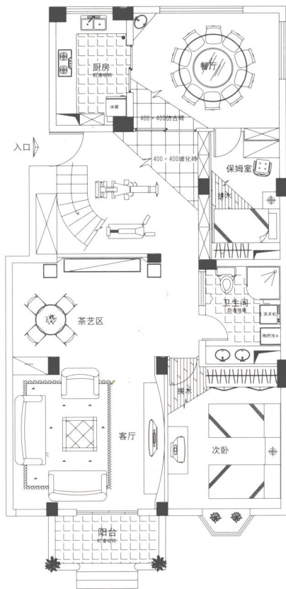
一层平面图
