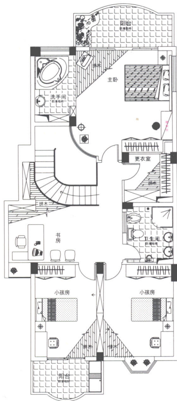
二层平面图
