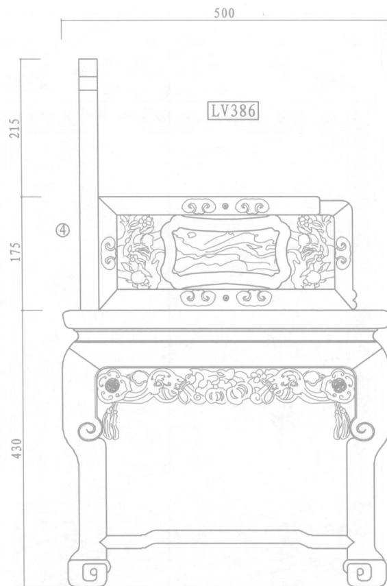
左视图 left view
