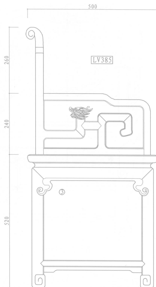
左视图 left view
