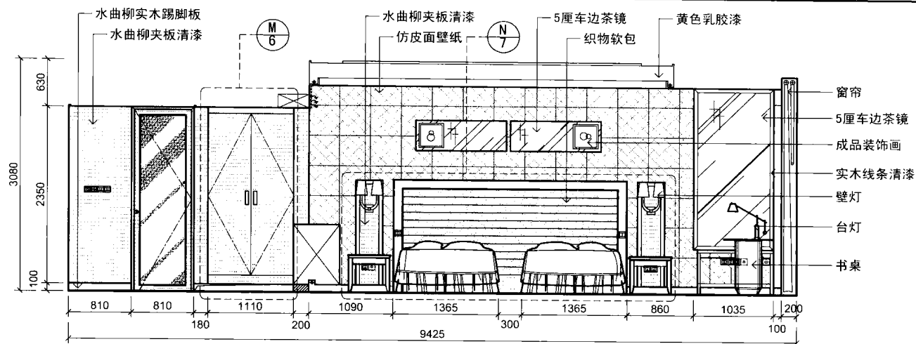
ELEVATION 展开立面图
