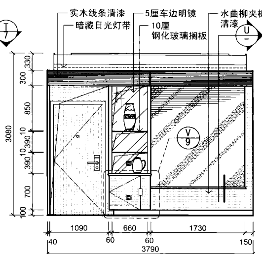
ELEVATION 立面图
