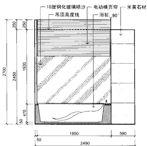
F ELEVATION 2 立面图
