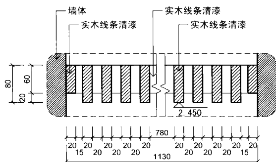
SECTION 剖面图
