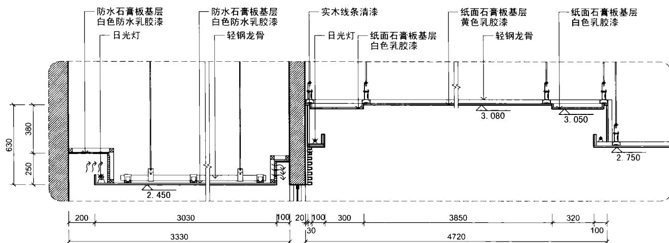
SECTION 剖面图
