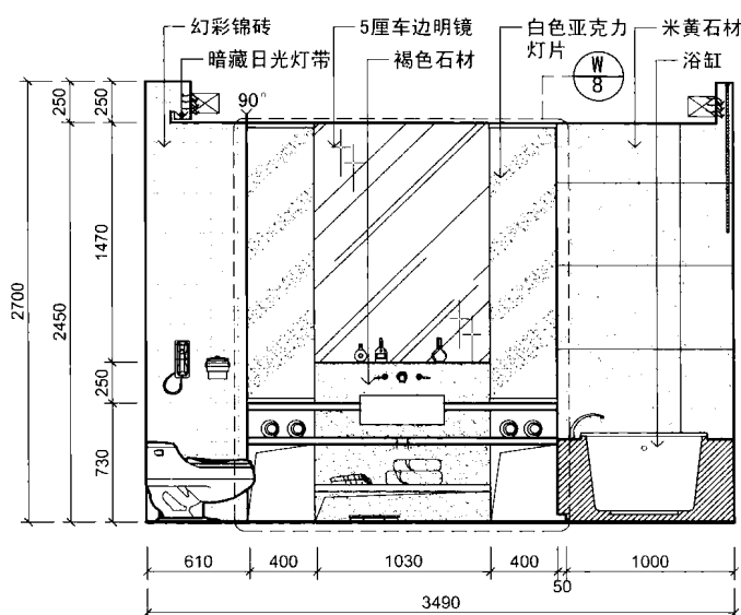
E 2 ELEVATION 立面图
