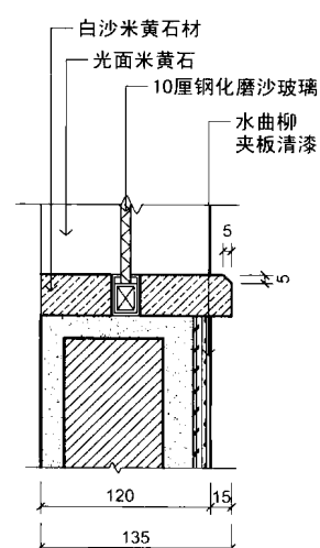
SECTION 剖面图
