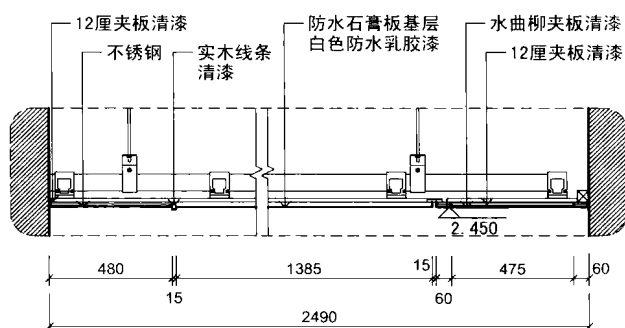
SECTION 剖面图
