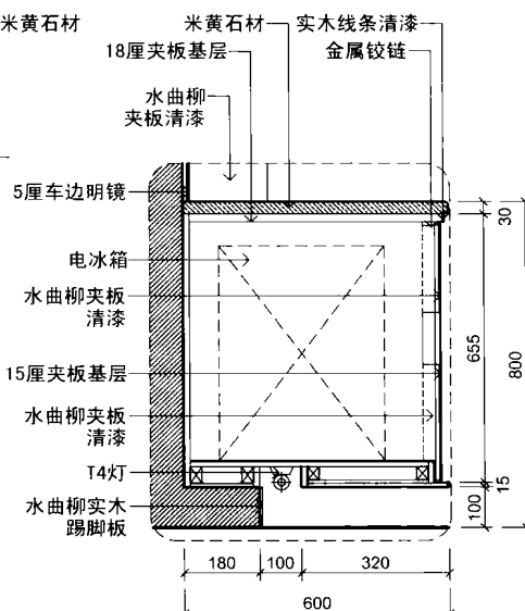
SECTION 剖面图
