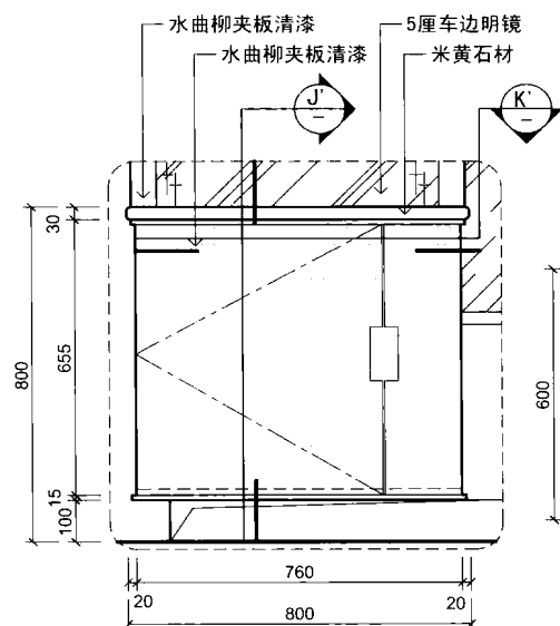
SECTION 剖面图
