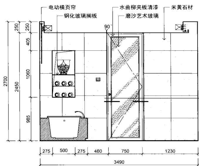
ELEVATION 立面图
