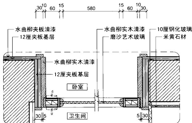
SECTION 剖面图
