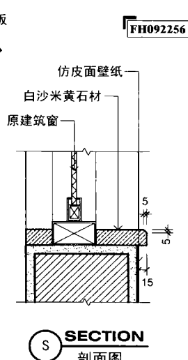
SECTION 剖面图
