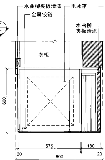
SECTION 剖面图
