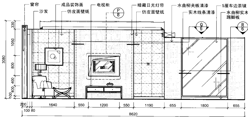
ELEVATION 立面图
