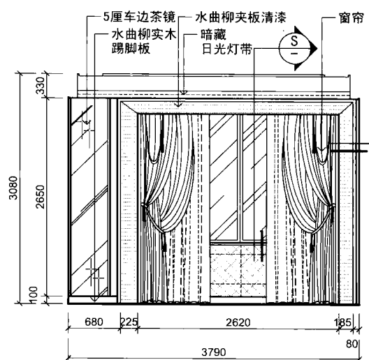
ELEVATION 立面图
