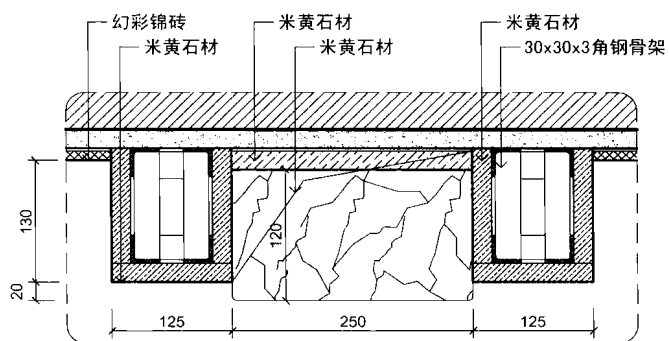
SECTION 剖面图
