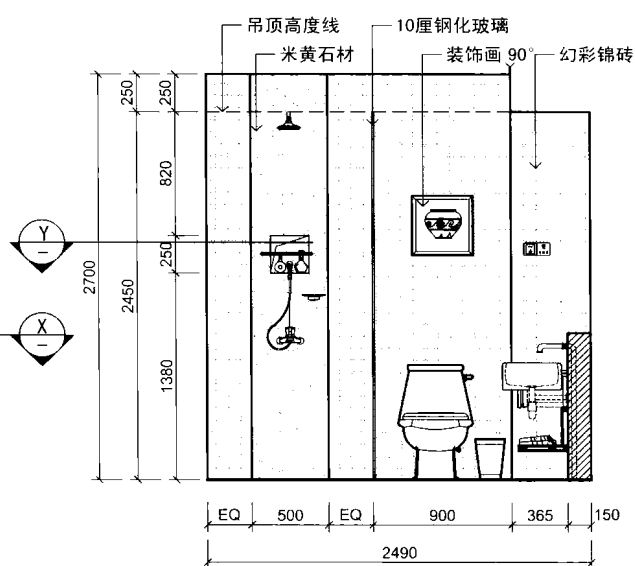
ELEVATION 立面图
