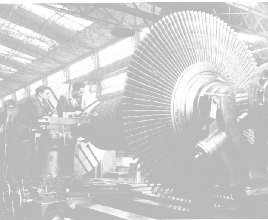
正在制造的高压透平机的旋转子。
