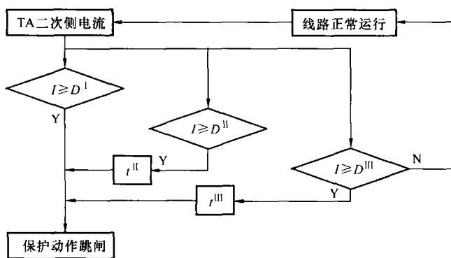
图 1-6 阶段式电流保护的工作流程
