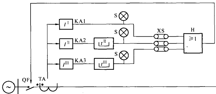
图 1-5 阶段式电流保护的逻辑框图
