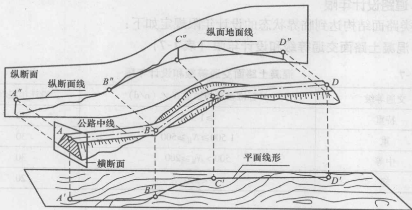
图 1-1 公路的平面、纵断面及横断面
