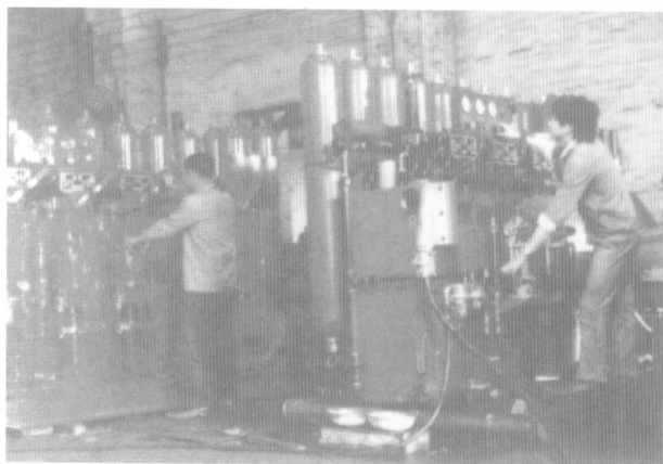
8月，由沙湾机械厂制造的钻井防喷液控装置，成为中国第一台自行设计和制造的钻井防喷液控装置
