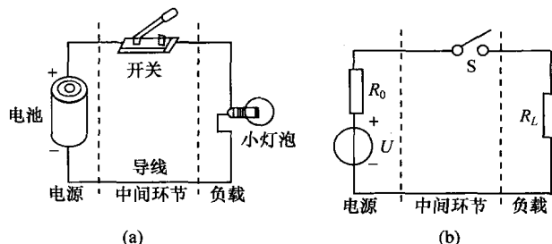
图 1.1.1 电路组成和电路模型
