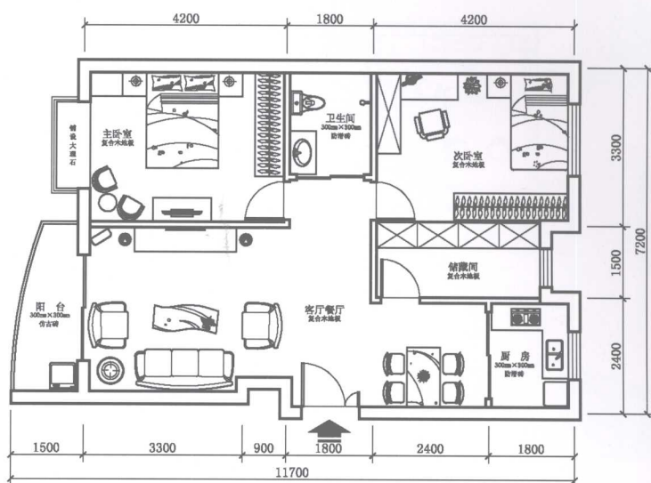
▲ 平面布置图
