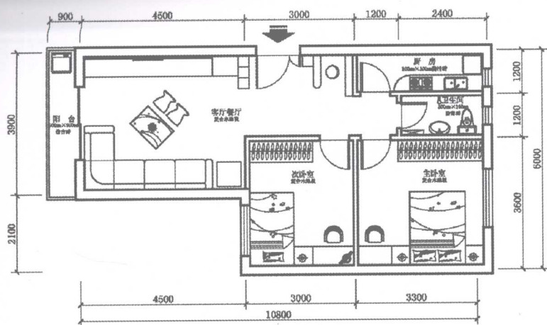
▲ 平面布置图
