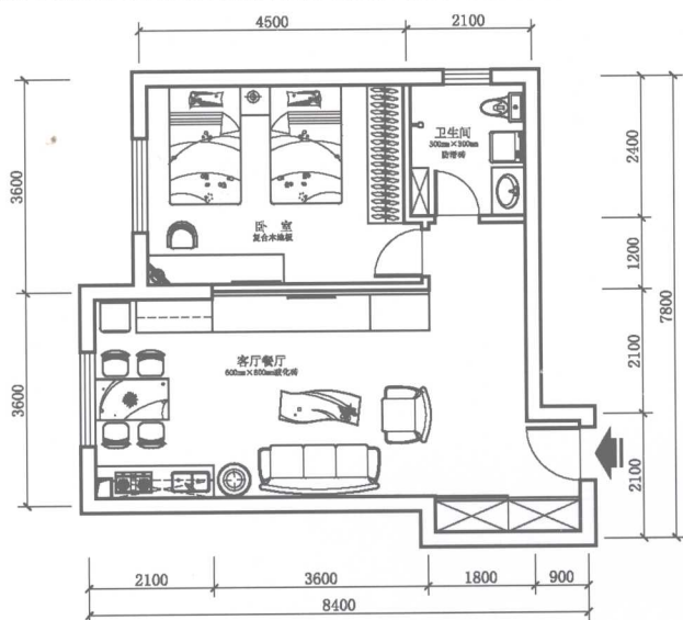
▲ 平面布置图
