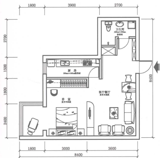
▲ 平面布置图
