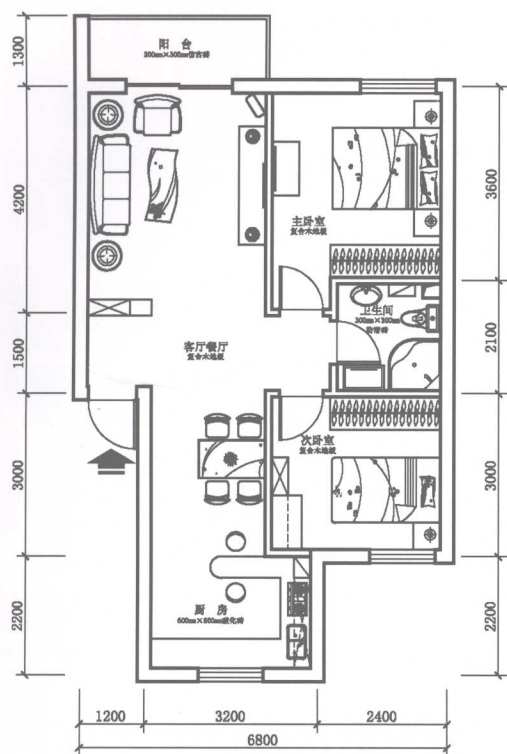
▲ 平面布置图
