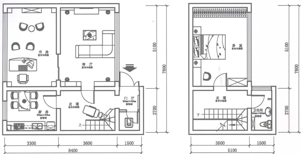
▲ 平面布置图
