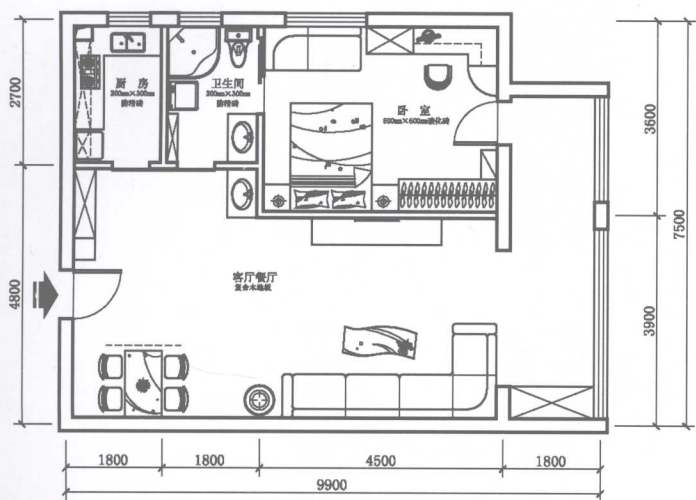
▲ 平面布置图
