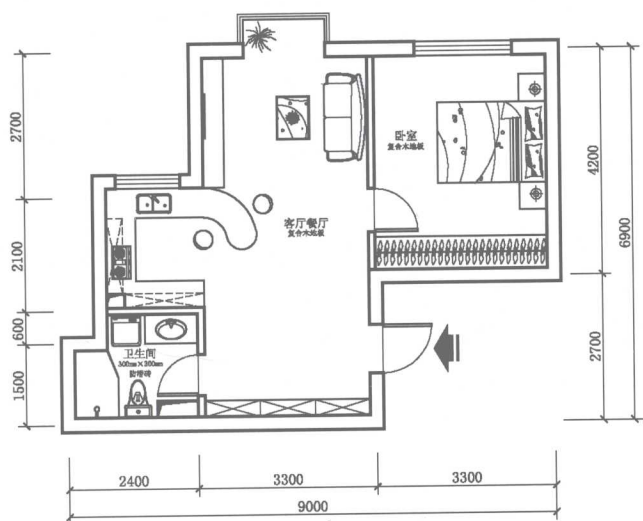
▲ 平面布置图
