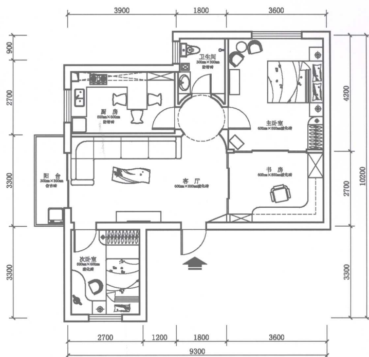
▲ 平面布置图
