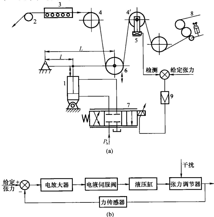
图 1-4 带钢恒张力控制系统
