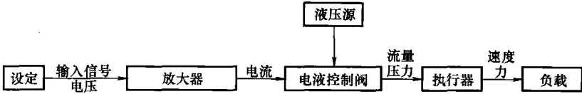
图 1-5 开环控制系统
