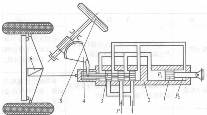
图 1-3 转向液压助力器原理图
