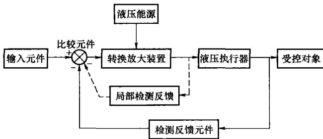
图 1-2 液压控制系统的组成
