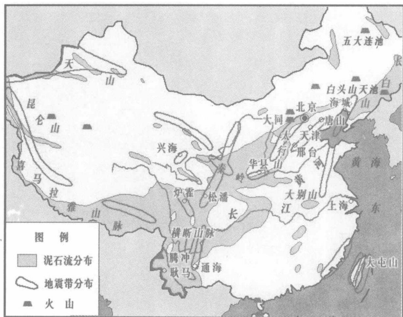
中国地震带分布图
