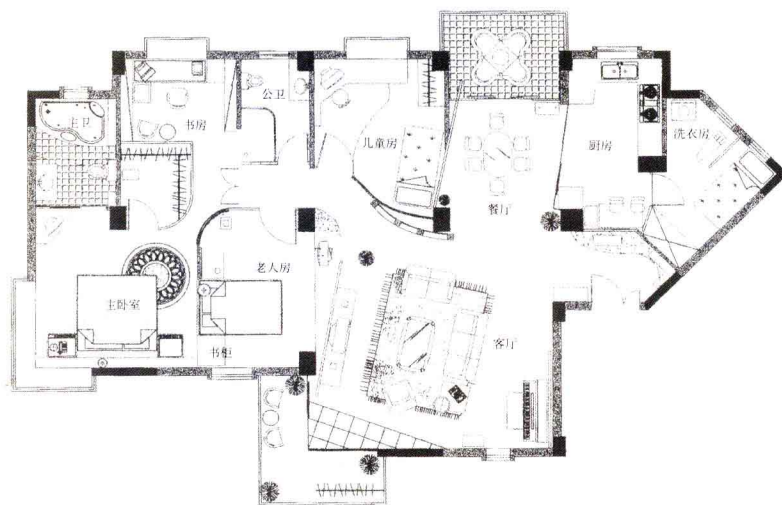
■ 平面图
