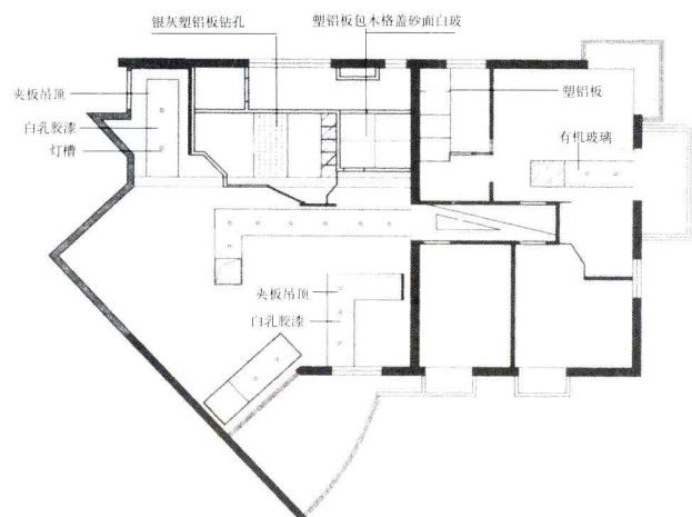
■ 天花图
