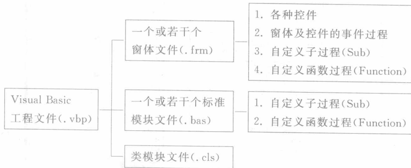
图 1-8 Visual Basic 应用程序中主要文件的关系
