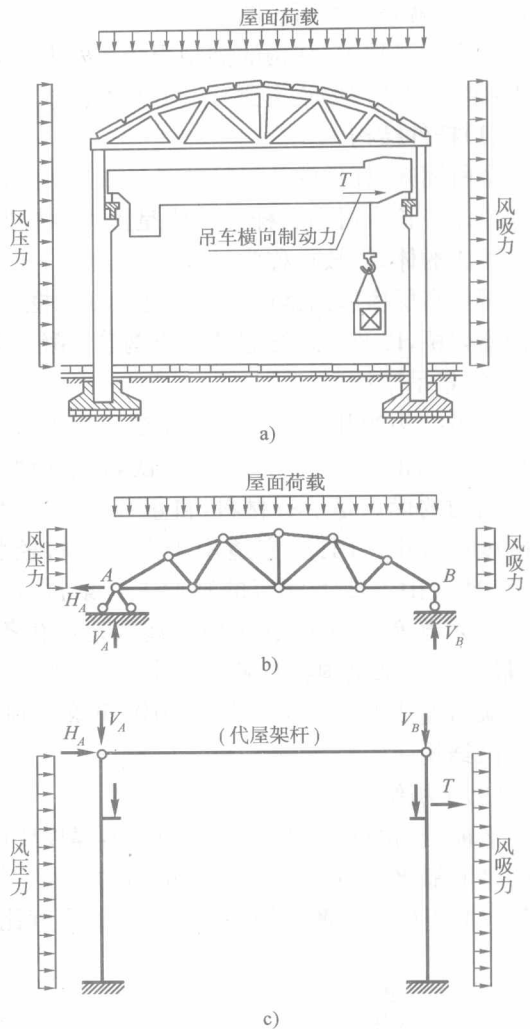
图 1-2 钢筋混凝土单层工业厂房计算简图
