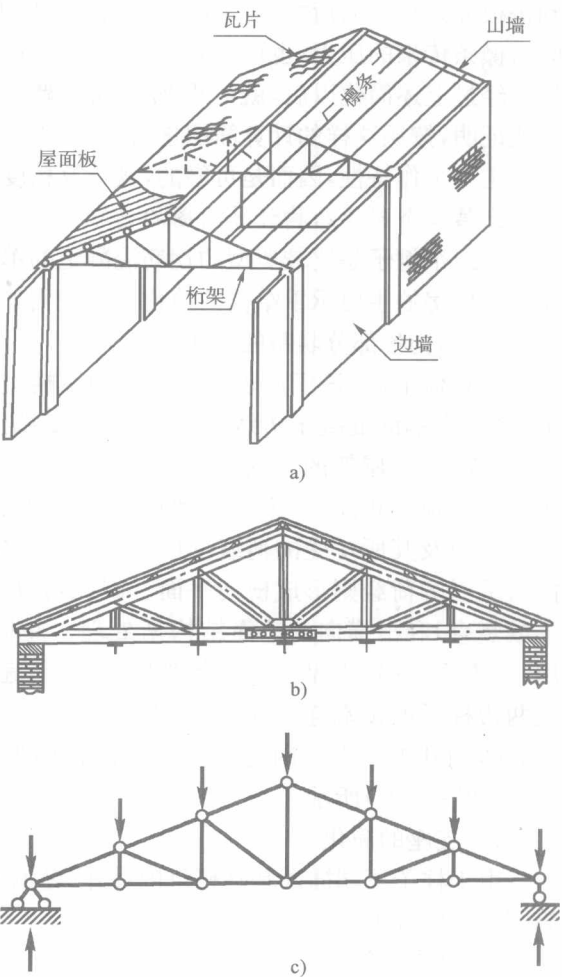
图 1-1 砖木结构民用房屋计算简图
