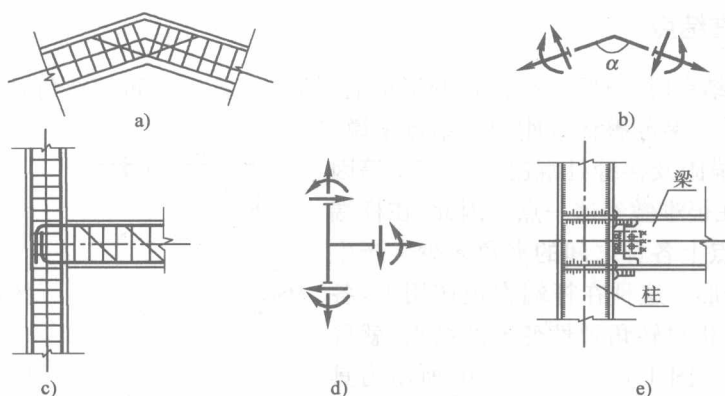
图 1-12 刚结点
