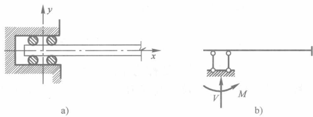
图 1-9 定向支座 a)定向支座构造;b)定向支座计算简图
