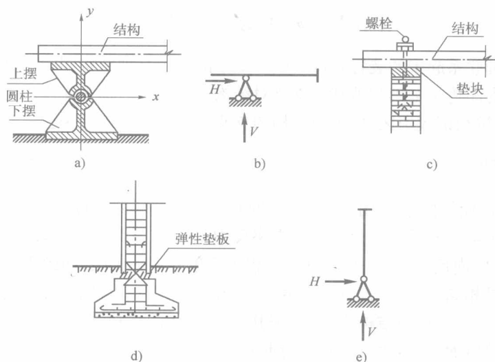
图 1-7 固定铰支座
