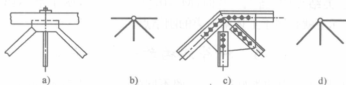
图 1-13 铰结点
