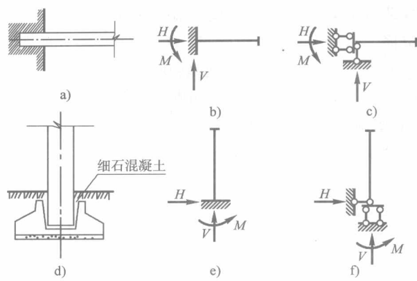
图 1-8 固定支座 a)固定支座构造;b)、c)计算简图;d)预制柱杯口基础;e)、f)计算简图
