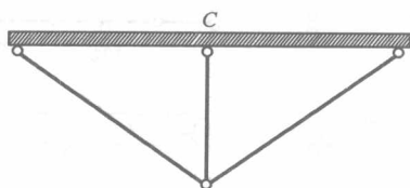
图 1-14 组合结点
