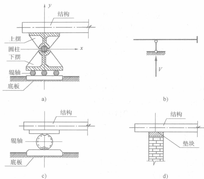
图 1-6 可动铰支座
