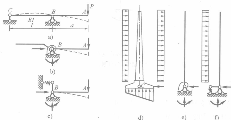
图 1-11 旋转弹性支座
