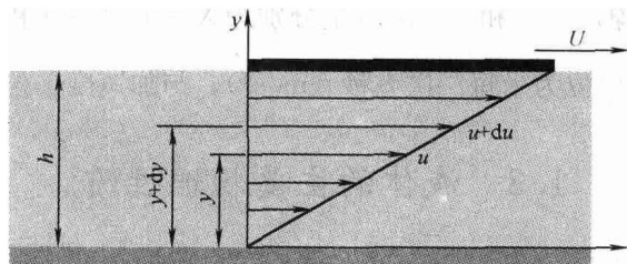
图 1-2 黏滞性实验
