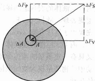
图 1-1 表面力
