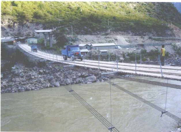
世界首座倒张式钢索吊桥——澜沧江甸尾桥
