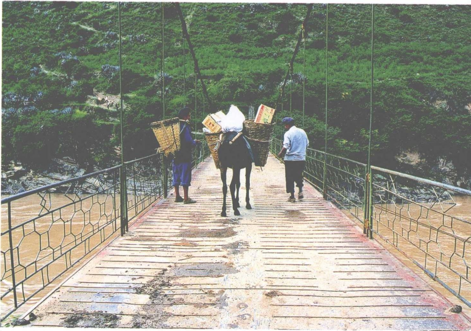
苏罗寨汽车吊桥
