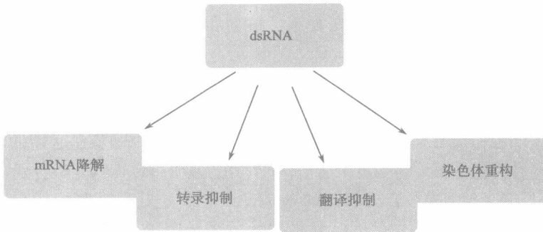
图 3 dsRNA 的分子调控分类 [19]
