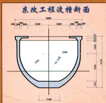
U型薄壳渡槽试验段
