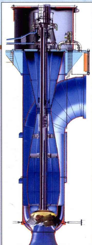
液压式全调节立轴抽芯式斜流泵模型
