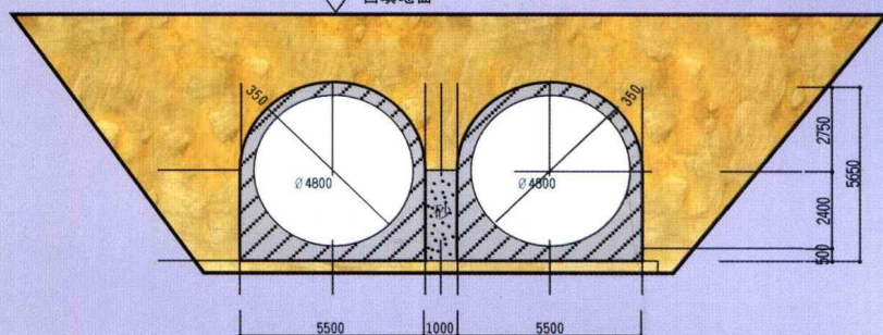
东深改造工程地下圆涵断面
