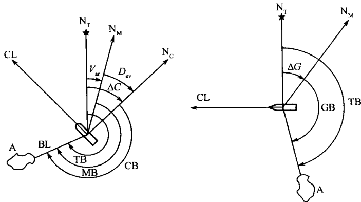
图 1-2 方位及其关系示意
