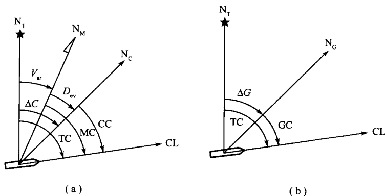
图 1-1 航向及其关系示意
