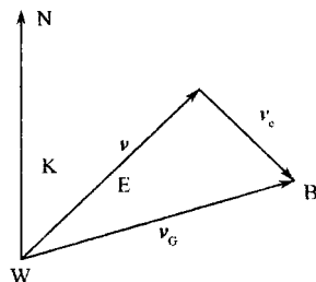
图 1-4 速度矢量三角形
