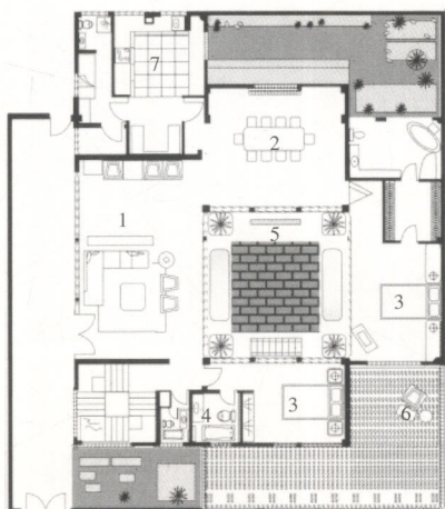
一层平面图
