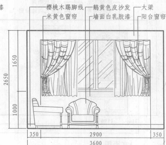
B立面图
