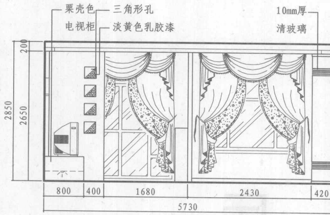
A立面图
