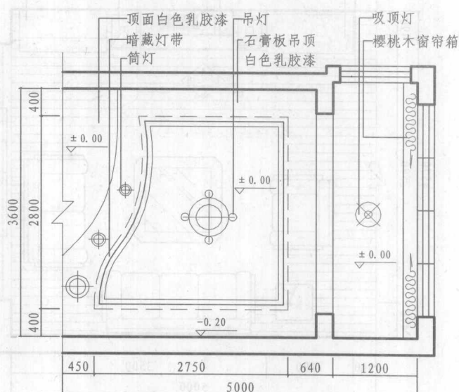
顶棚图
