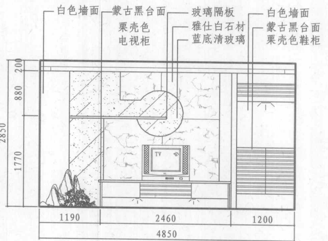
D立面图
