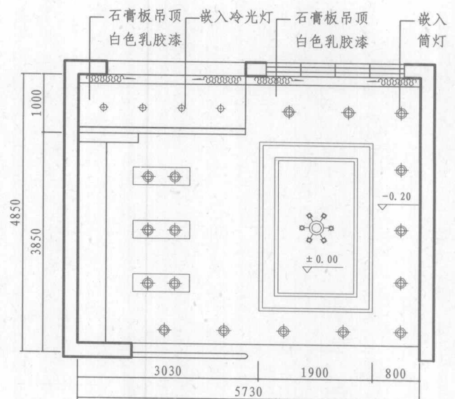
顶棚图
