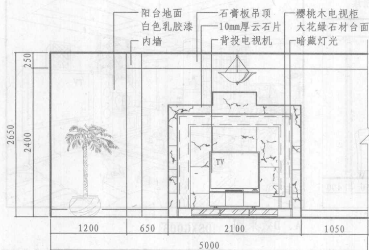
C立面图
