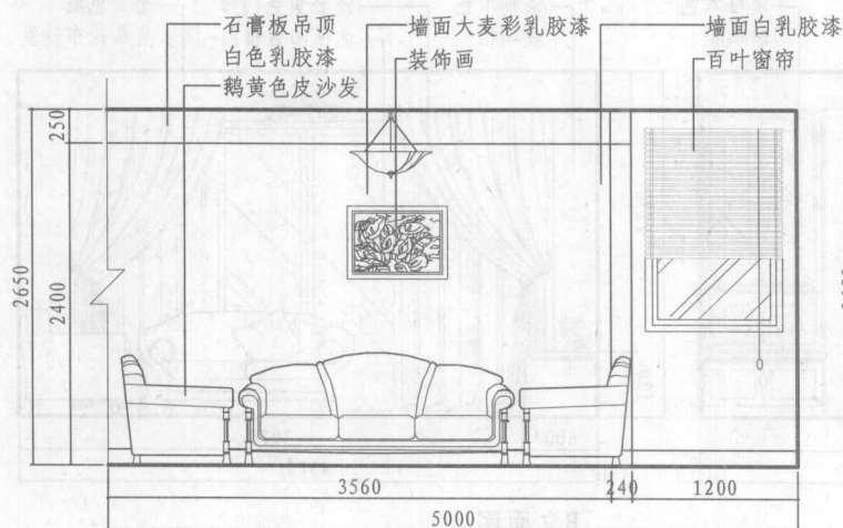
A立面图
