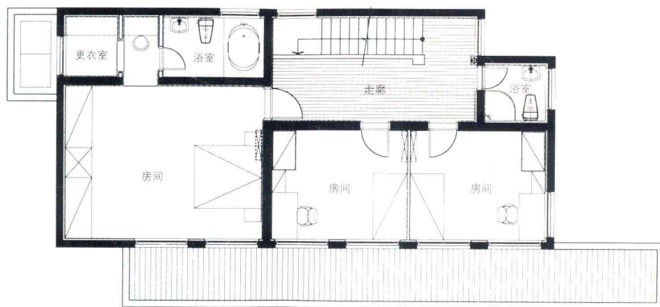
二楼平面图
