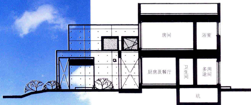
横剖面图
