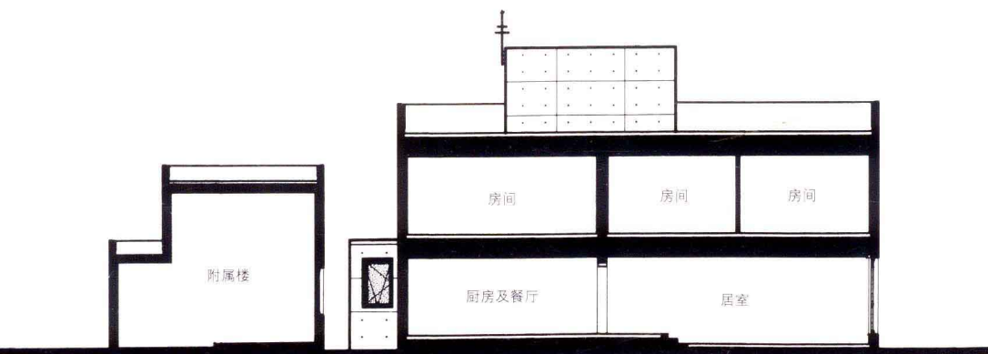
纵剖面图
