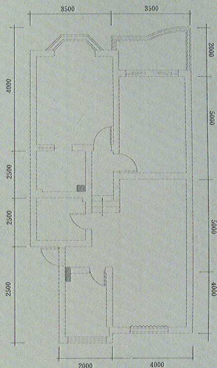
原结构平面图
