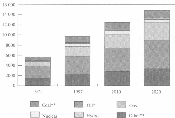
图 1-1 2020 年前世界一次能源供应量预测
