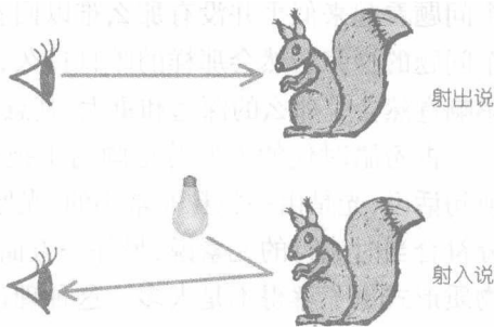
图 1.3 视觉成像的几种理论
