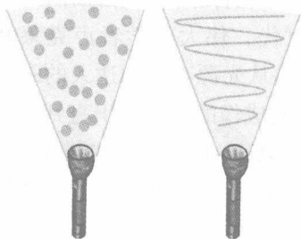
图 1.4 光的微粒说和波动说
