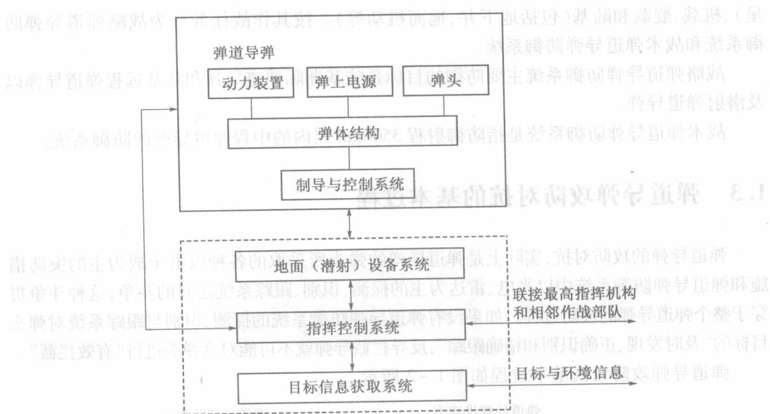
图 1-1 弹道导弹武器系统基本组成图
