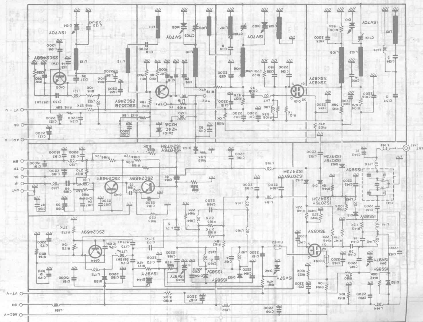
调谐器电路图
