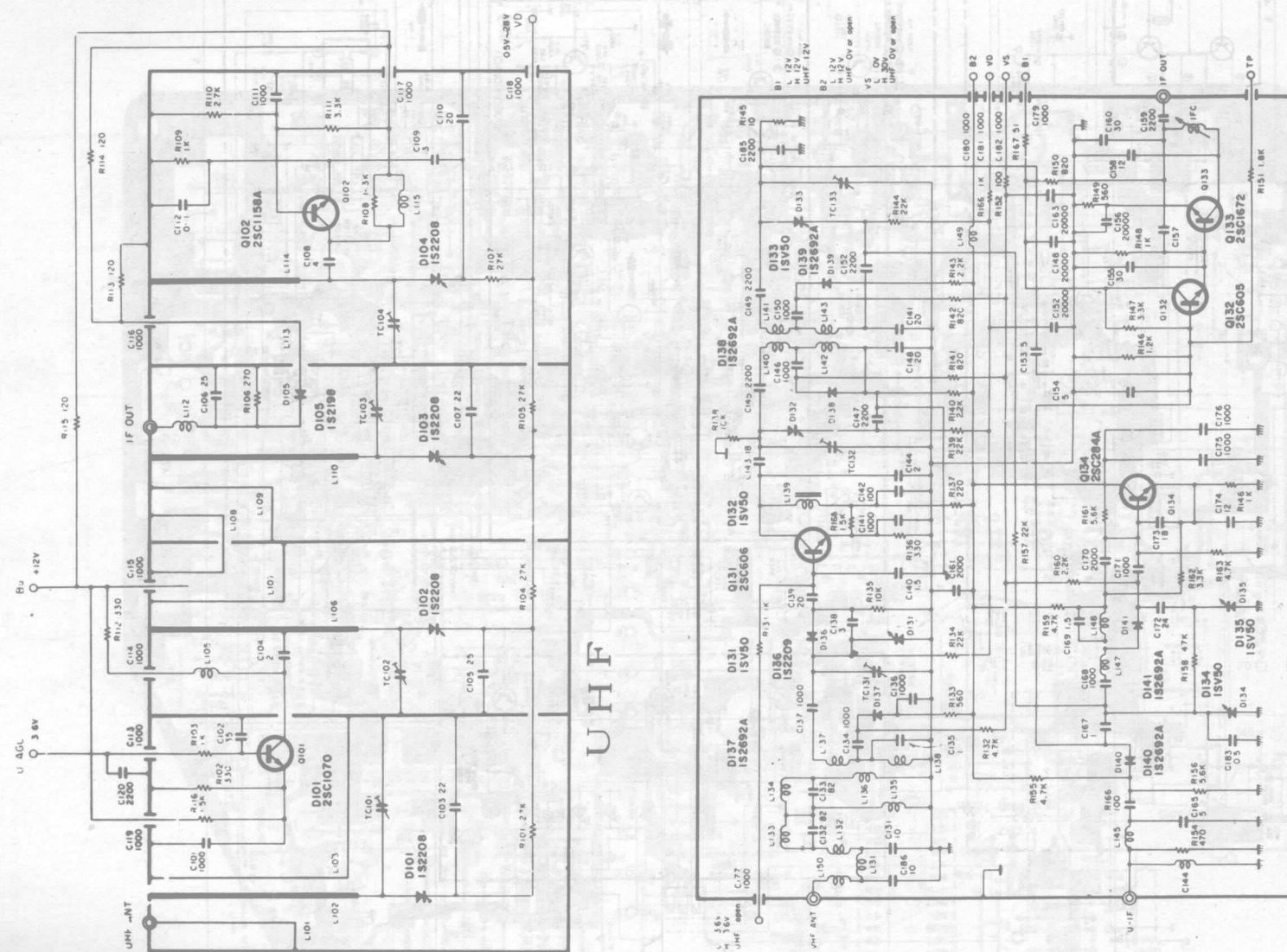
调谐器电路图
