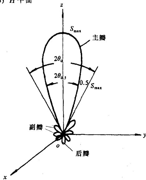
图 1-6 天线波瓣参数
