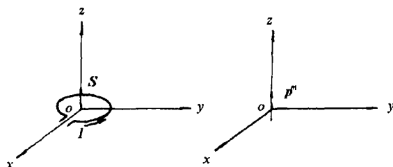
图 1-3 小电流环与磁矩
