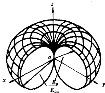
图 1-4 电基本振子空间方向图
