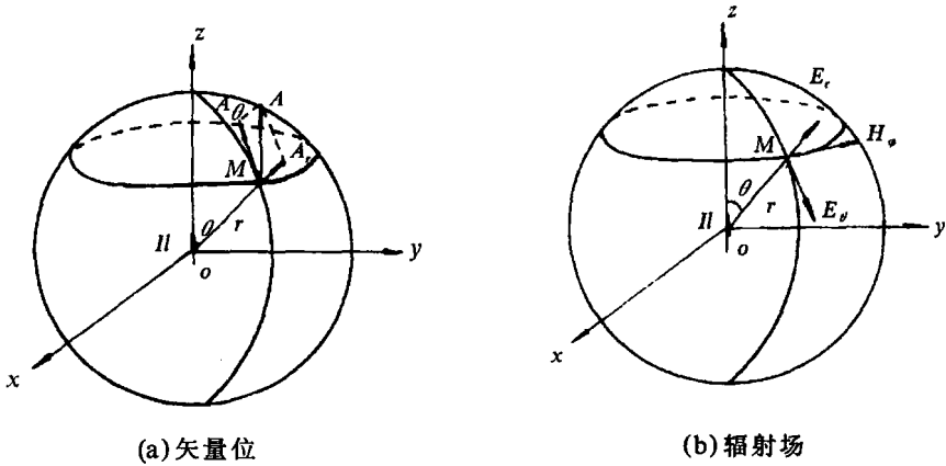
图 1-1 电基本振子的矢量位与辐射场分量
