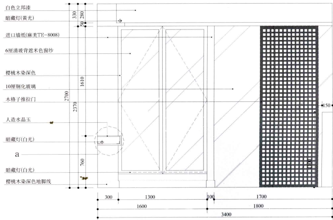
◆主卧室 A 立面图
