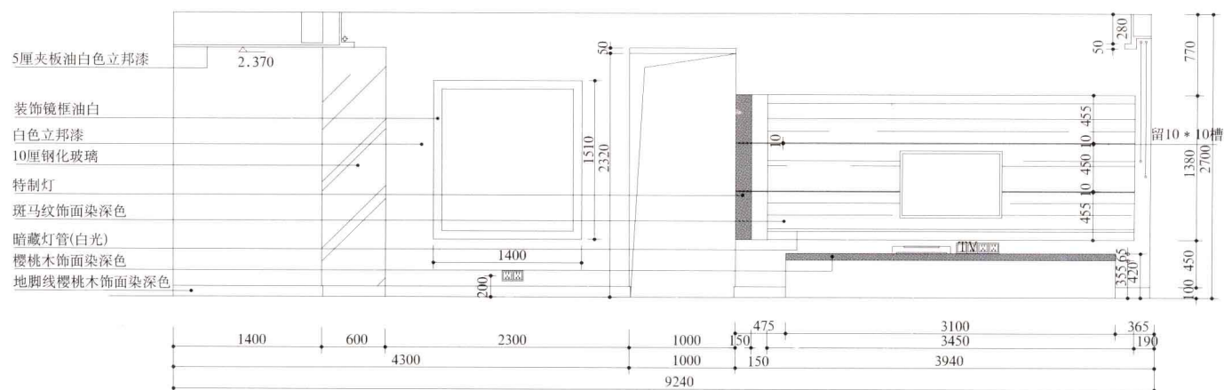
◆客厅 A 立面图
