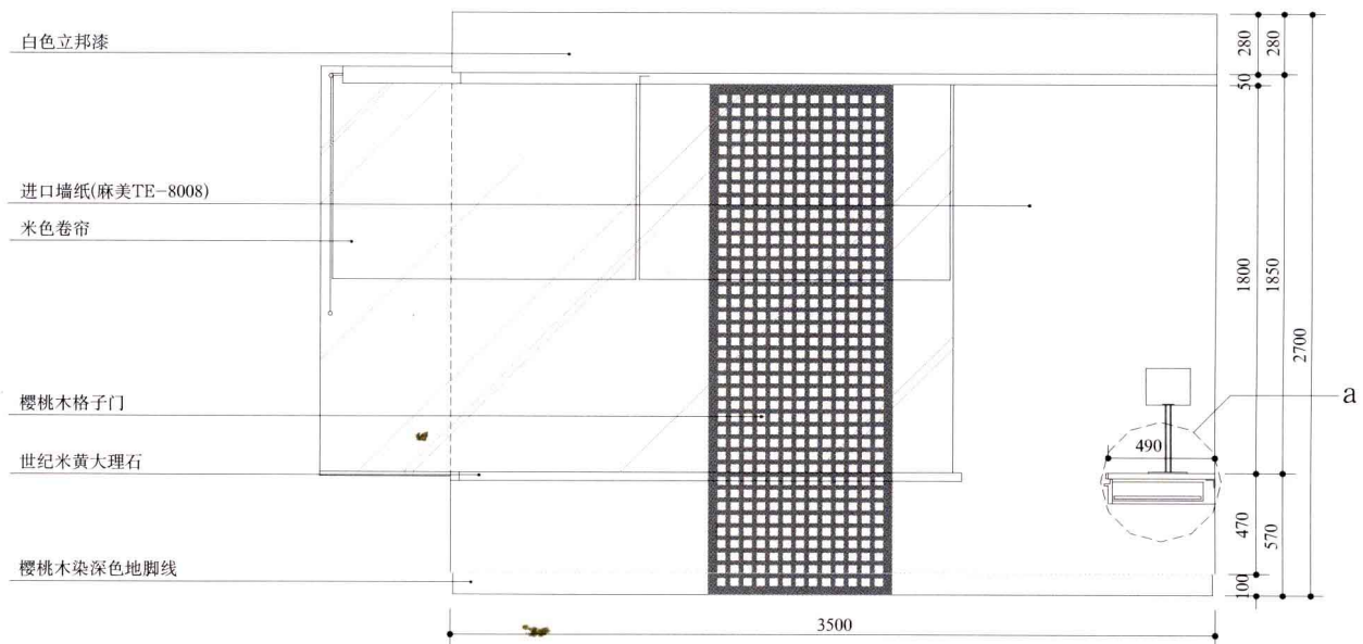
◆ 主卧室 C 立面图
