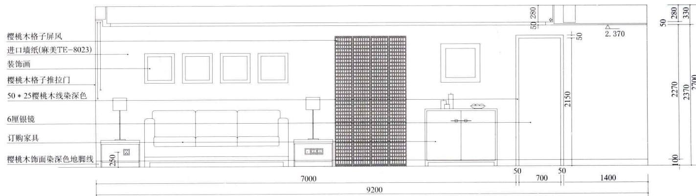
◆客厅 B 立面图
