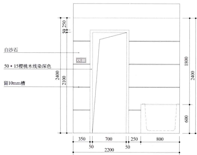
◆ 主卫 A 立面图
