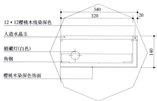
◆ 主卧室 C 立面大样图 a
