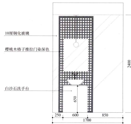
◆ 主卫 B 立面图
