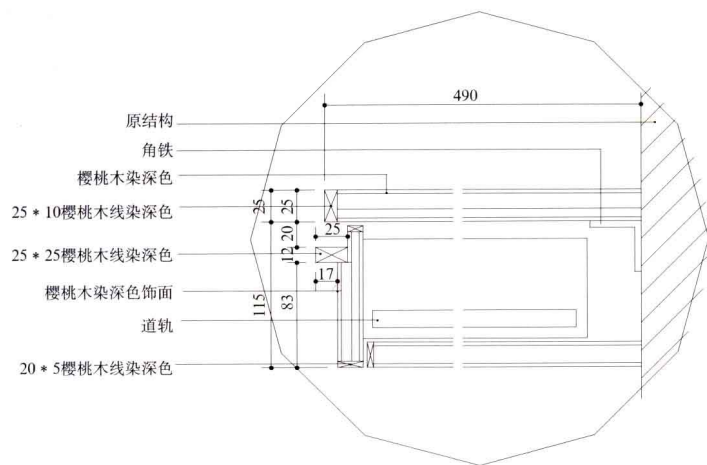
◆主卧室 A 立面大样图 a
