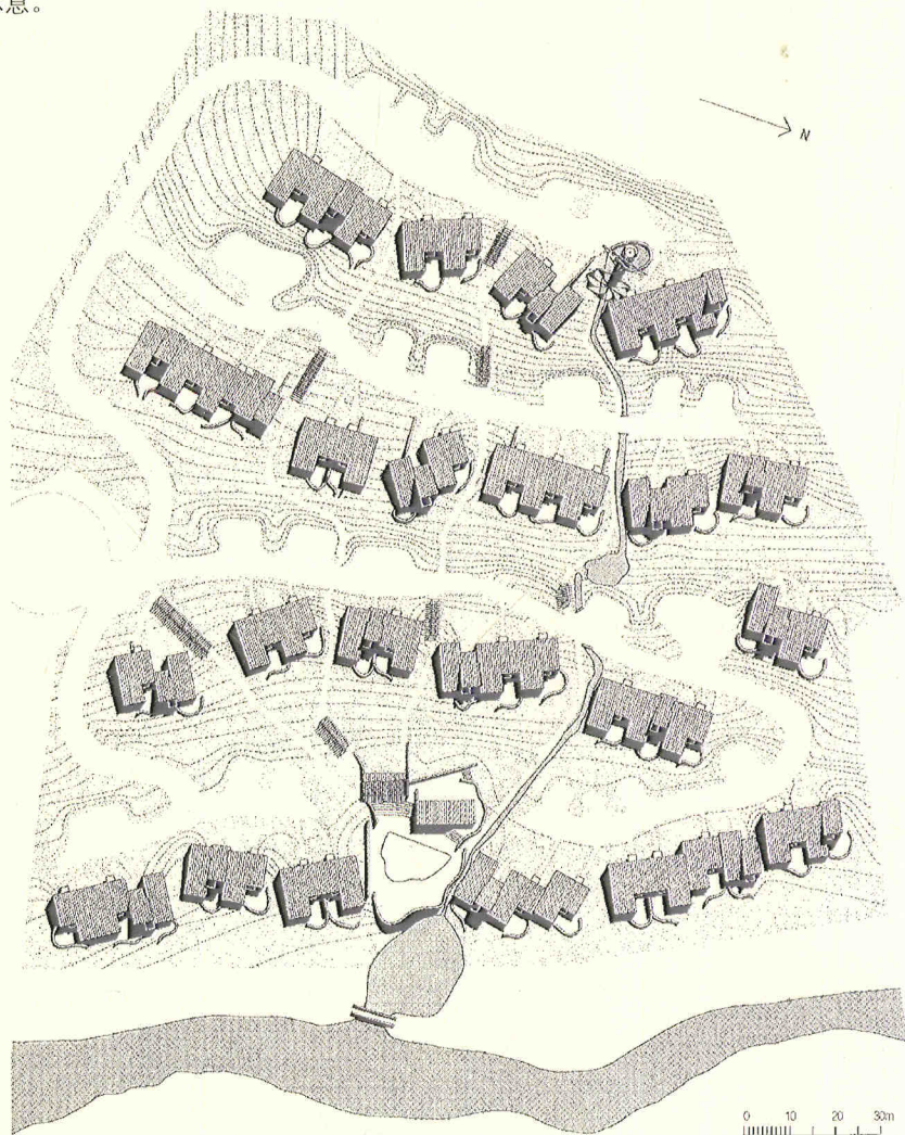
总平面图
