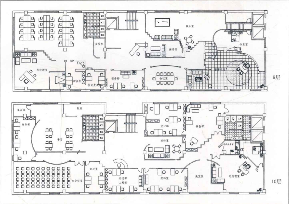
平面图
