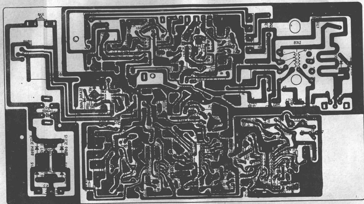
印制版图
