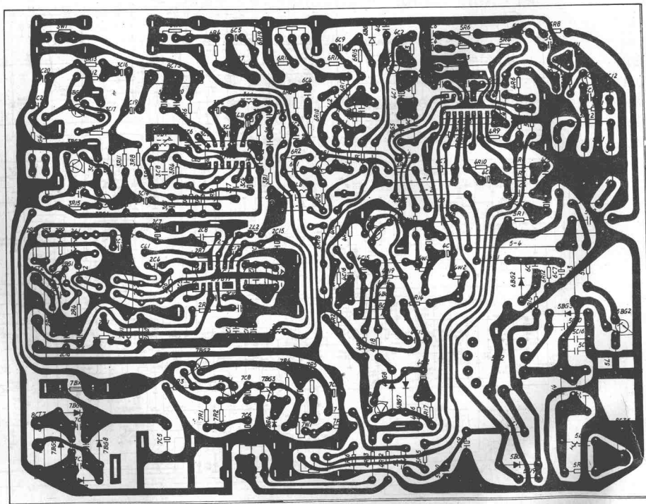
印制版图
