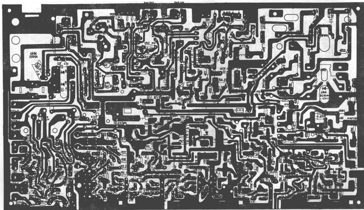
印制版图
