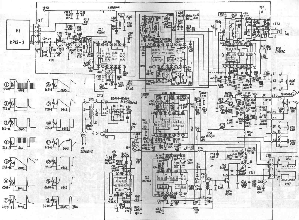
电原理图
