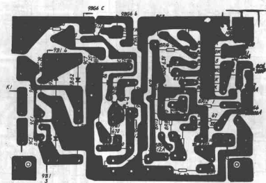
图 2. 电源及功放印制电路板图
