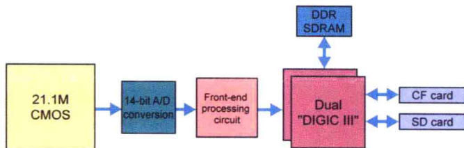
佳能 EOS-1DsMark3 采用了 14 位 A/D 模拟数字转换芯片和两个“DIGIC”DSP 处理芯片，并安装了大容量的 DDR 内存
