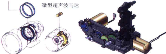
佳能摄影镜头内的超声波马达
