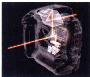
尼康数码单反相机的光学结构图
