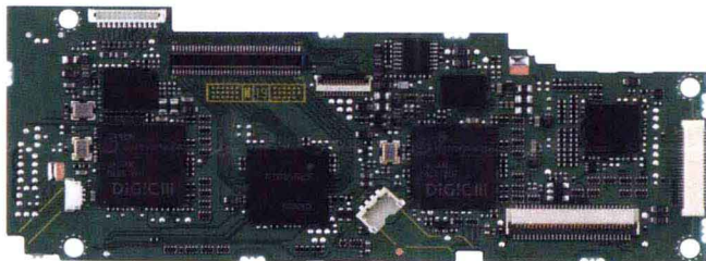
佳能 EOS-1DsMark3 采用了两颗 DSP 数字处理芯片 (DiGiC 芯片)，可以 5 张 / 秒的速度连拍 56 张 2200 万像素分辨率数码相片
