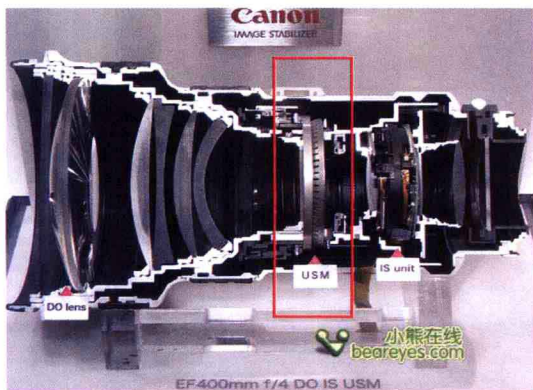
佳能将 USM 超声波马达安装在了摄影镜头里面（红框内就是 USM 超声波马达）
