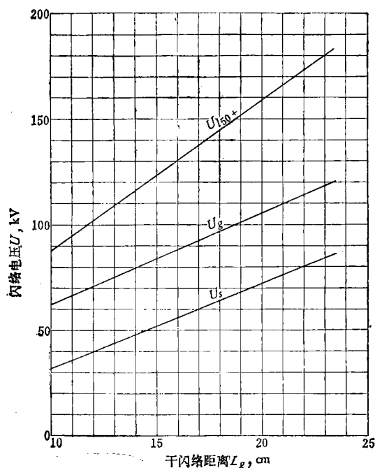
图27-2-4 针式绝缘子闪络电压曲线
