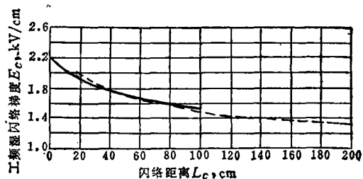
图27-2-7 普通伞裙绝缘子垂直安装时
