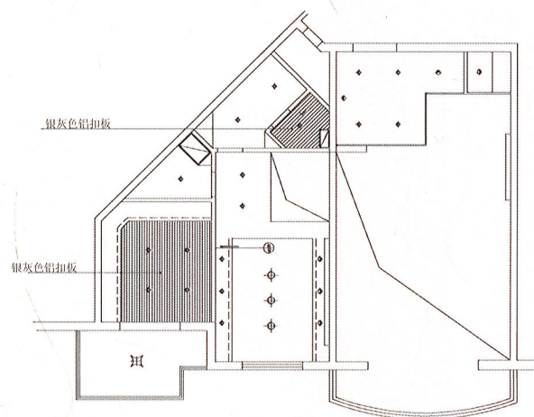
■ 一层天花图
