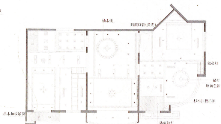
■ 一层天花图
