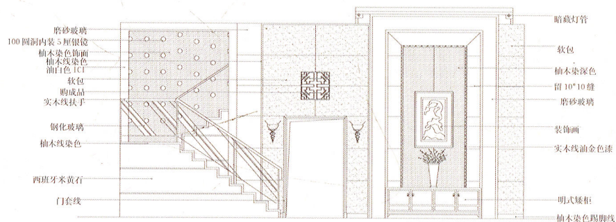
■ 客厅立面图
