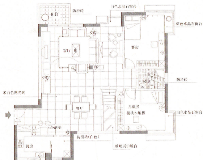
■ 一层平面图
