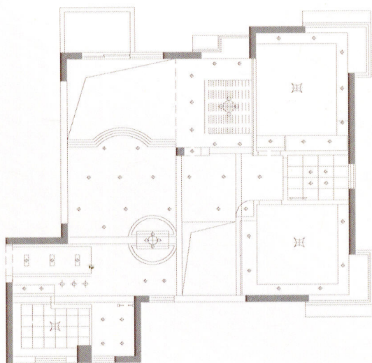
■ 一层天花图
