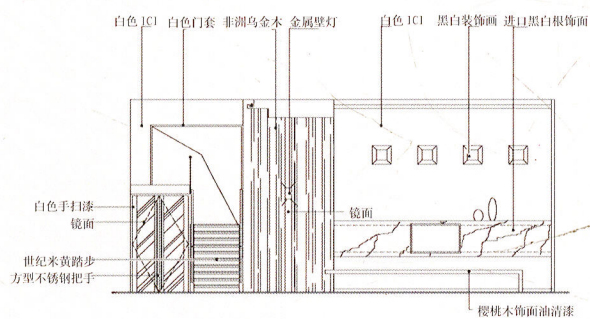
■ 客厅立面图
