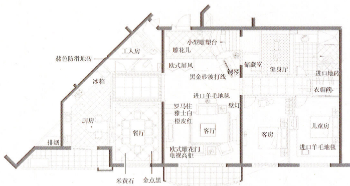
■平面图
