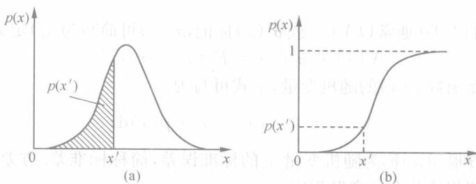
图 0.2.2 连续型随机变量 X 的概率密度函数(a)和分布函数(b)
