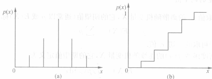
图 0.2.1 离散型随机变量 X 的概率函数(a)和分布函数(b)
