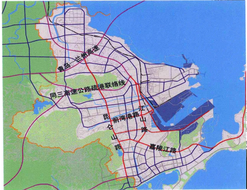
黄岛城区“四横两纵”路网示意图
