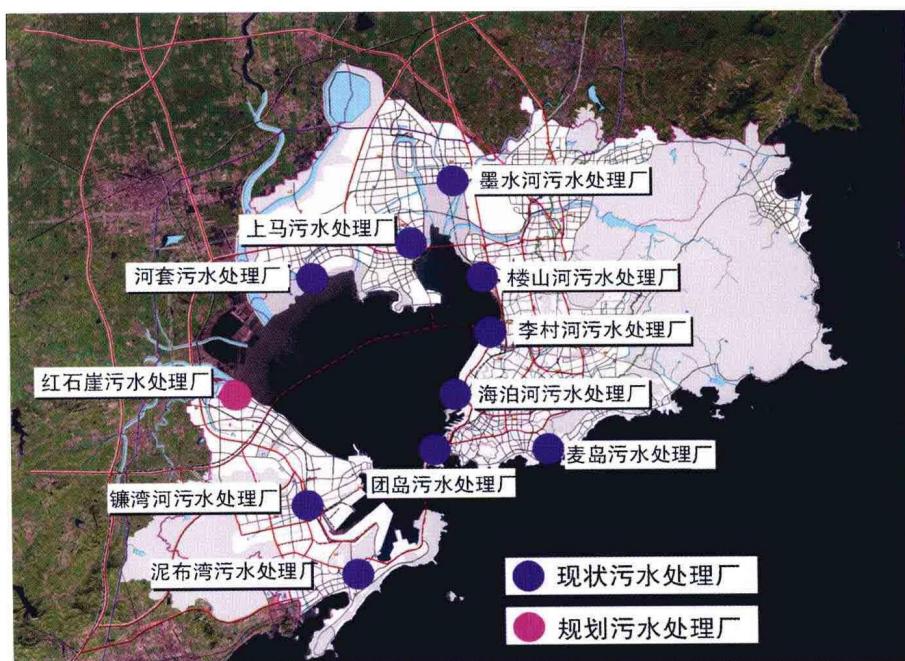
污水处理系统规划示意图
