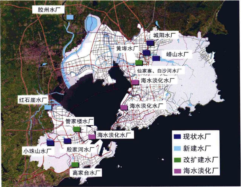
城市净水厂规划示意图
