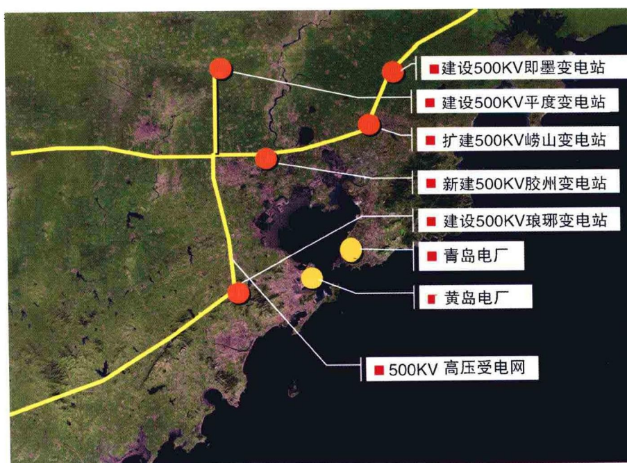
环湾区域500千伏变电站规划示意图
