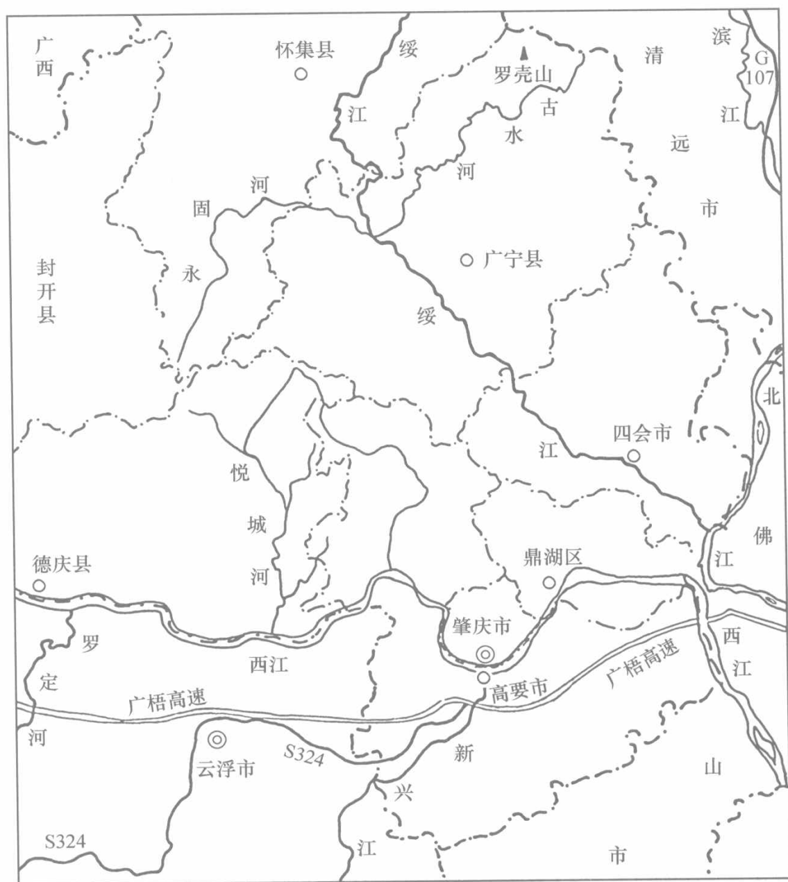
图二 广宁县、四会市地理位置示意图
