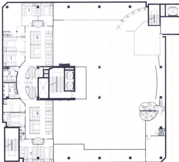
夹层平面图 The Middle Story Plan
