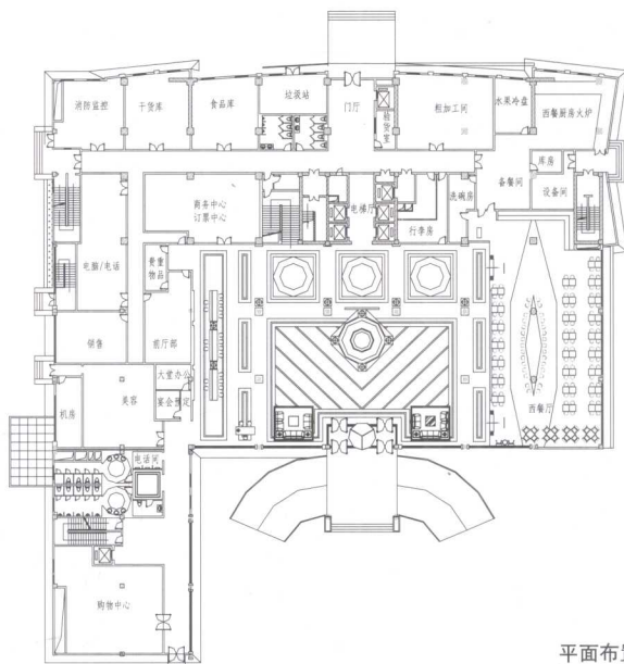
平面布置图
