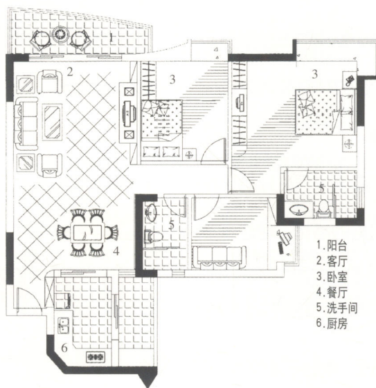
平面图
