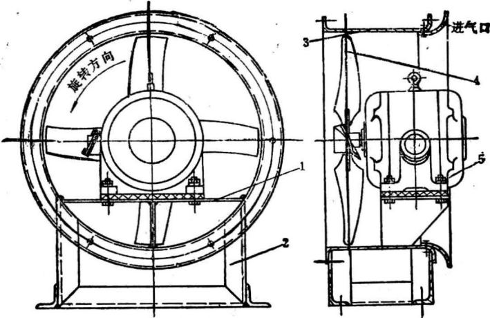
图7-1-3 低压轴流通风机
