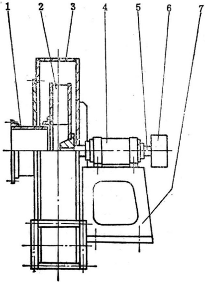
图7-1-2 高压离心通风机
