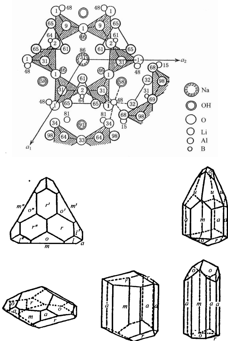
图 2-1 托玛琳的晶体结构
