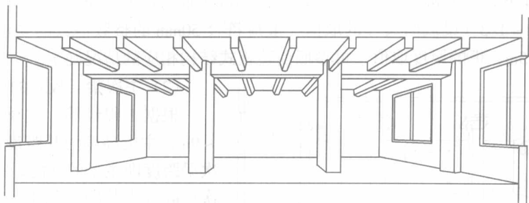
图 1-4 主次梁梁板式楼、屋盖结构示意图
