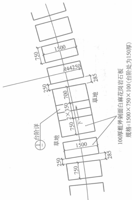
园路铺装平面图
