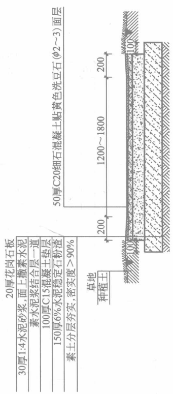
1-1剖面图
