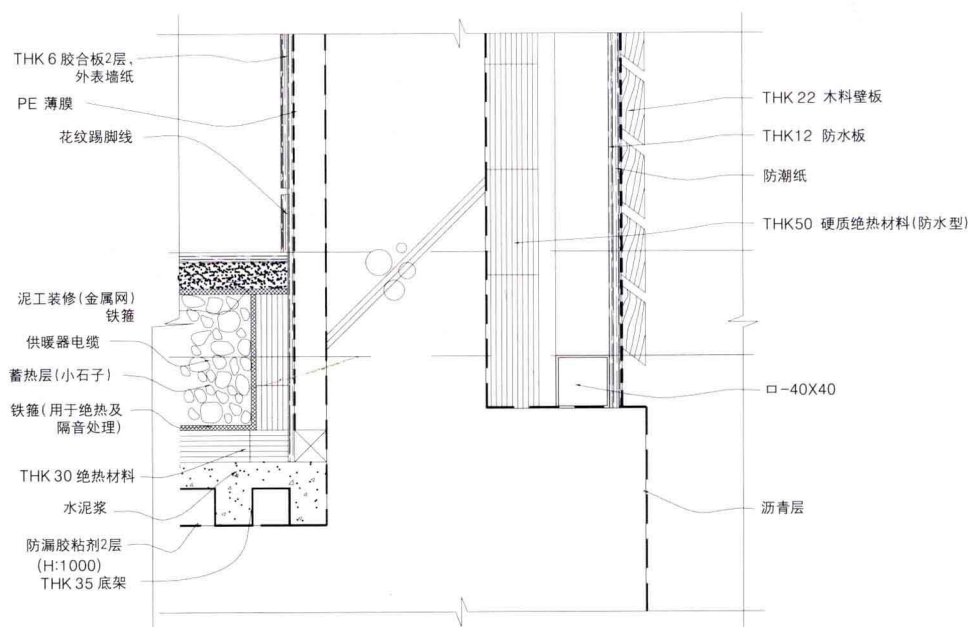
B - IV 部分详图
