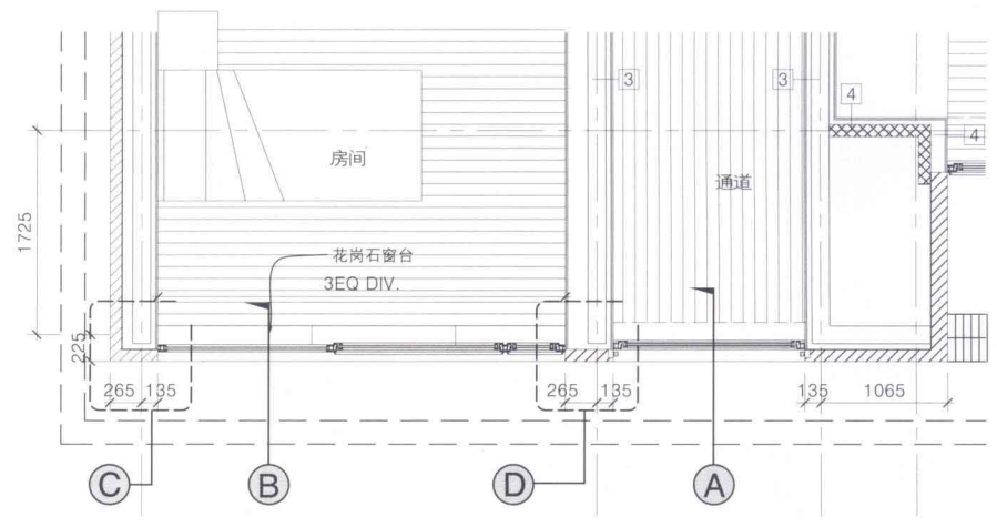
卧室 2 部分扩大的平面图
