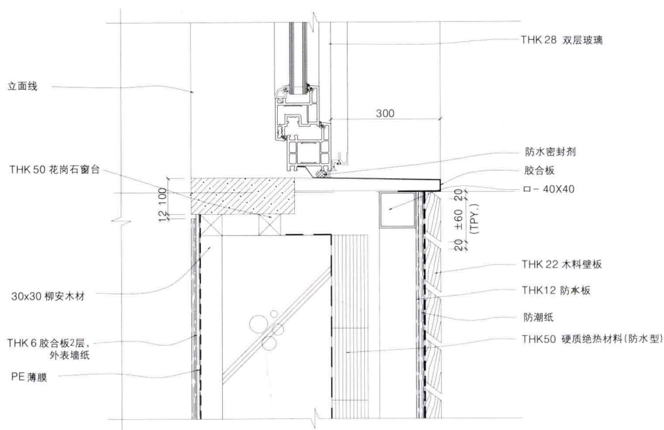
B - III 部分详图
