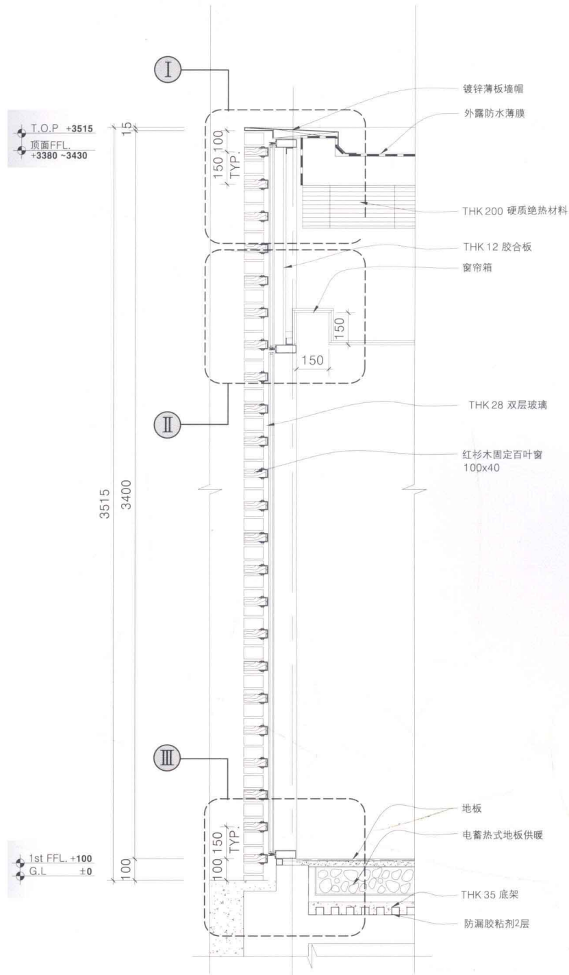
庭院侧通道的外墙断面图(A部分)
