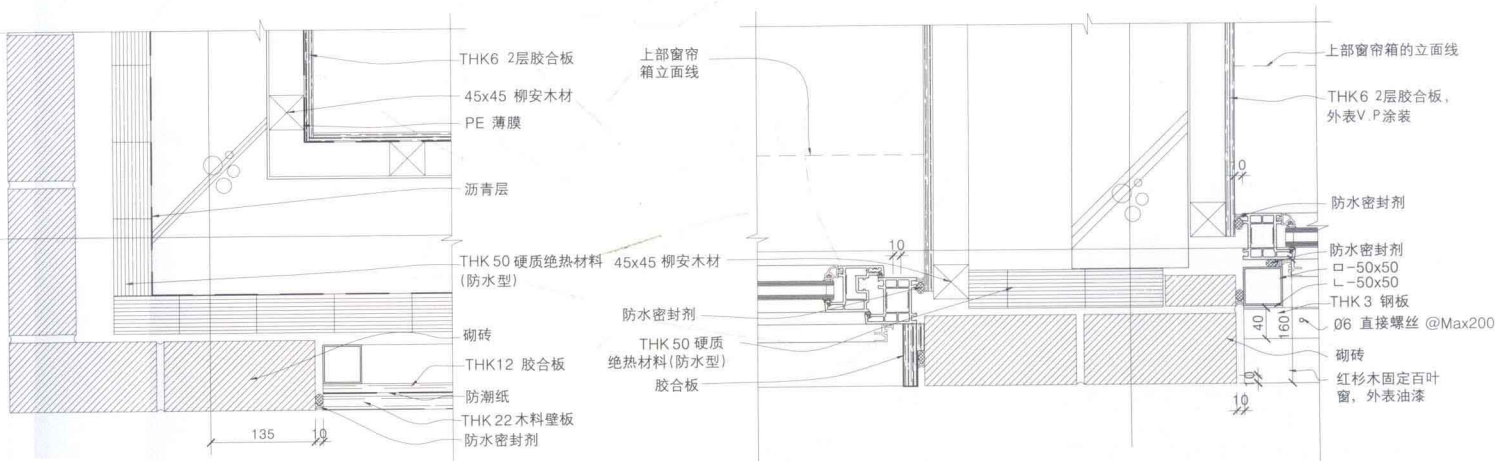
卧室和通道间墙壁的处理详图(D部分)
