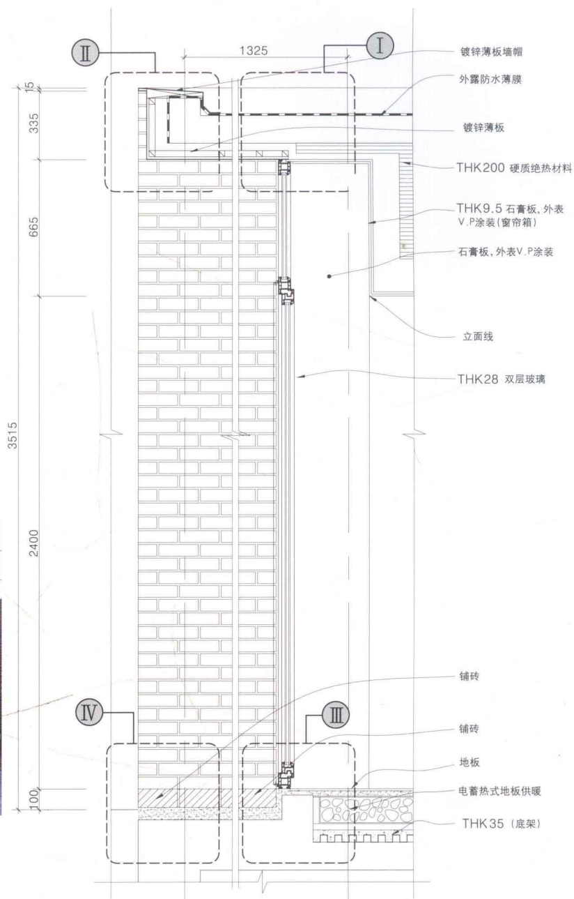
玻璃墙断面图(F部分)
