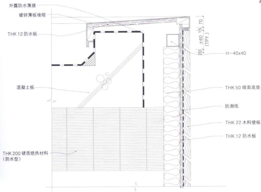
庭院侧卧室(书房)的断面详图
