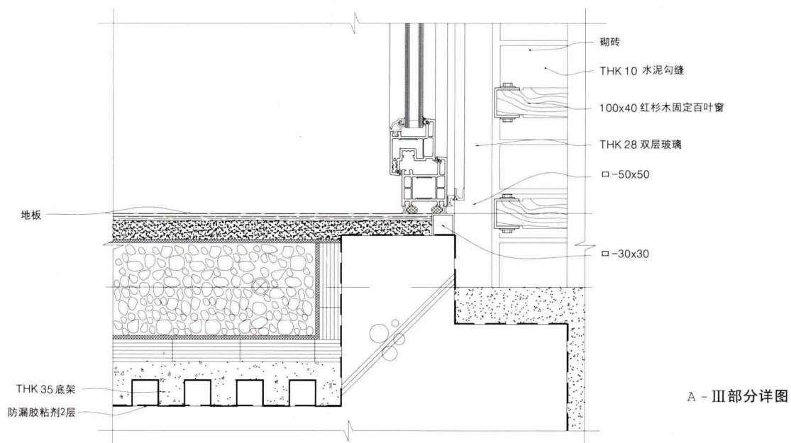
庭院侧通道部分外墙断面详图
