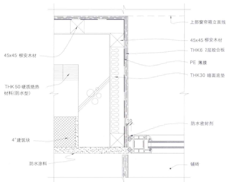
E部分的平面扩大图
