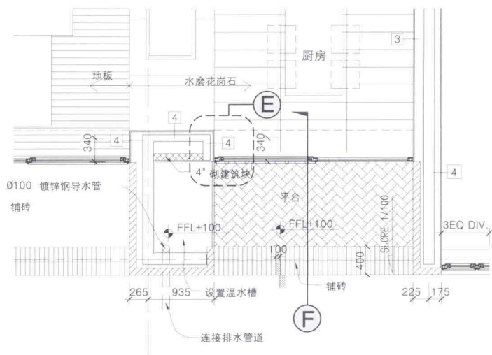
平台的平面扩大图
