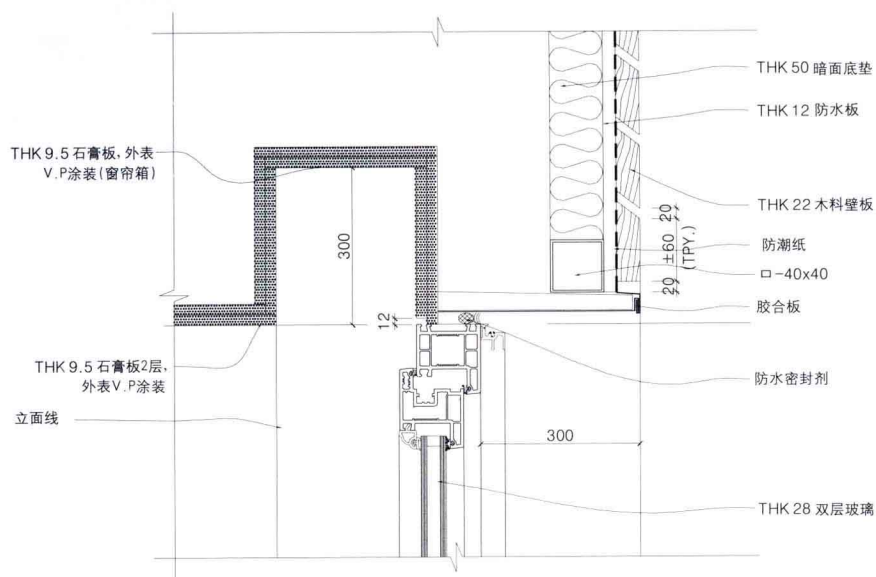
B - II 部分详图
