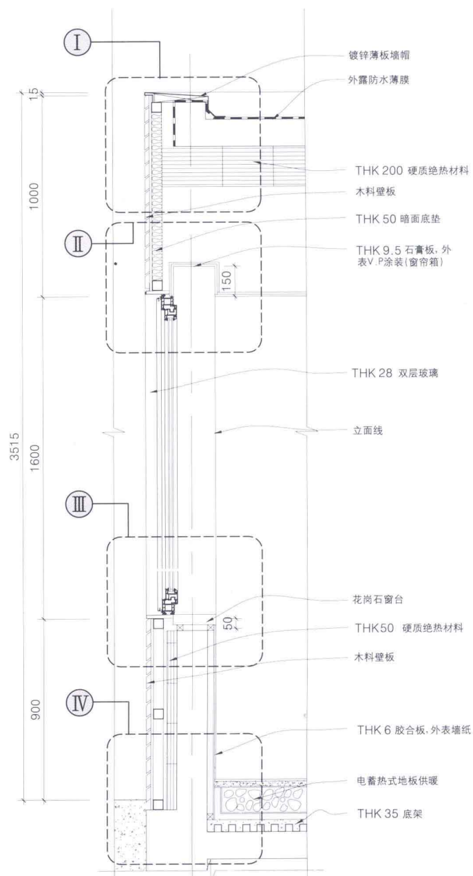
庭院侧卧室(书房)外墙断面图(B部分)
