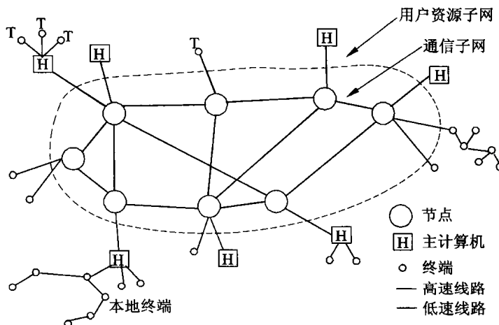
图 1-1 资源子网与通信子网
