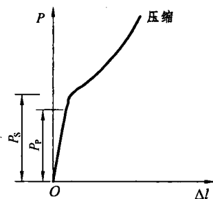
图 2.7 低碳钢压缩曲线
