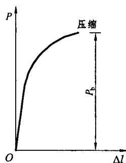
图 2.9 铸铁压缩曲线
