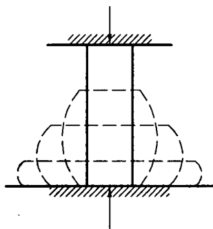
图 2.6 低碳钢压缩时的鼓胀效应
