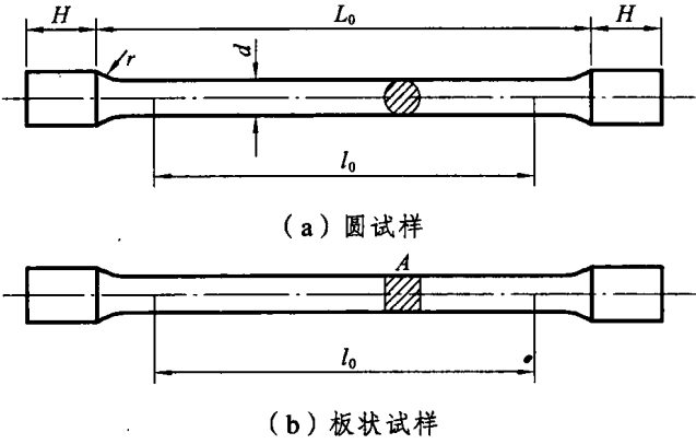
图 2.1 金属材料试样
