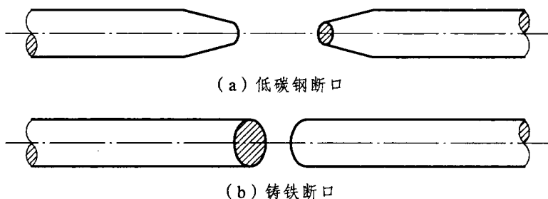
图 2.3 拉伸试样断口形状
