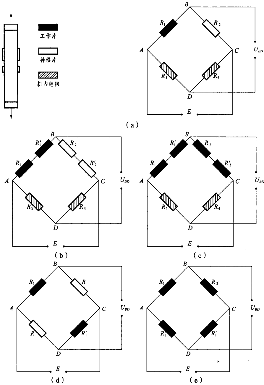
图 2.11 几种常见的组桥方式
