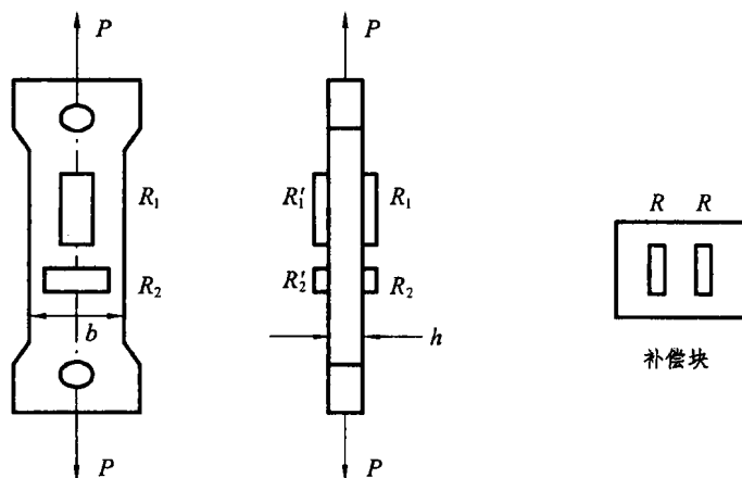
图 2.10 拉伸试件及布片图
